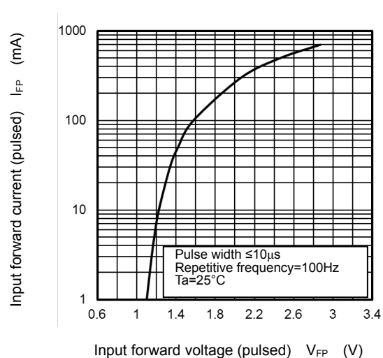
I_{FP} - V_{FP}
