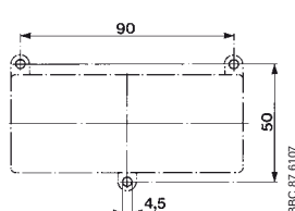
VB6(7), VBC6(7) VB6A(7A), VBC6A(7A)
