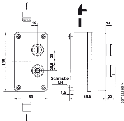
Dimension diagram DRB6 / DRB7
